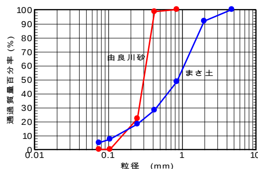
図1 試料の粒度分布
