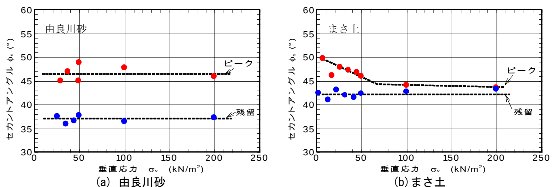
図4 セカントアングルと垂直応力の関係
