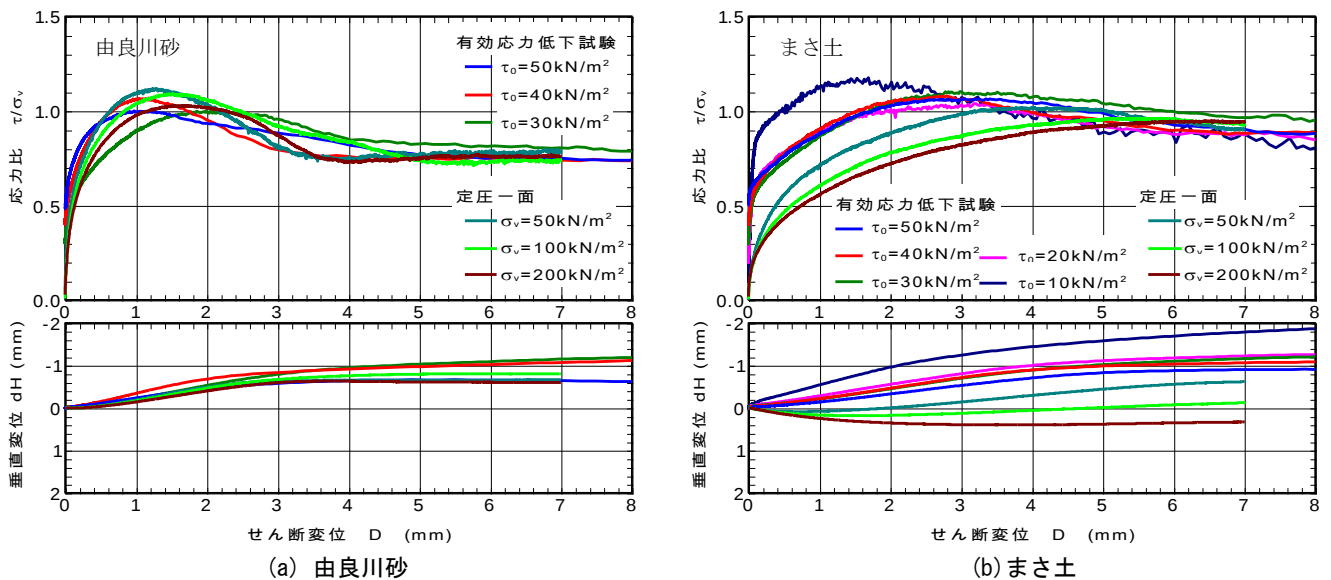
図3 せん断変位に対する応力比および垂直変位の変化
