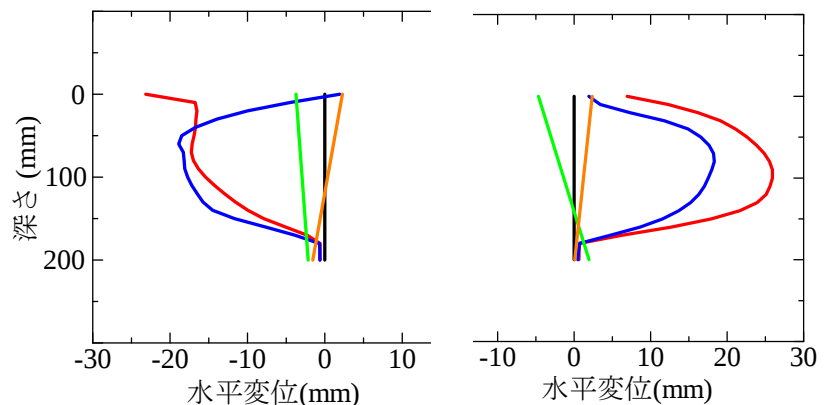
図4 水平変位
