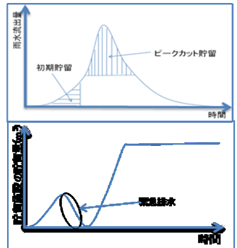
図2:実時間制御の概念図
