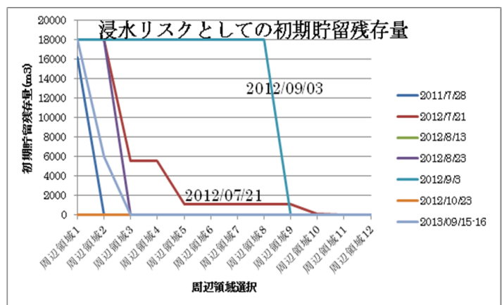
図3:ピークカット事例での浸水リスク（最大値選択）
