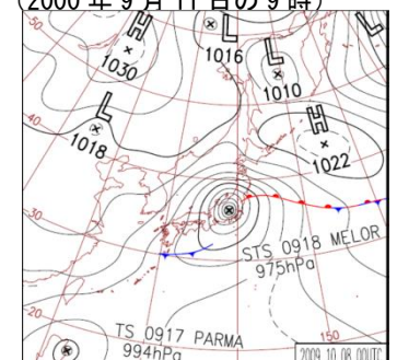
図 - 4 ②に該当する典型事例
