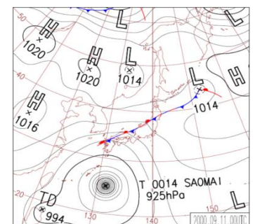
図 - 3 b) - ①に該当する典型事例
