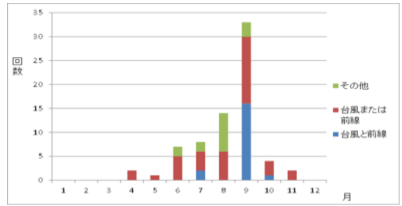
図 - 7 気圧配置による分類の月別の傾向
