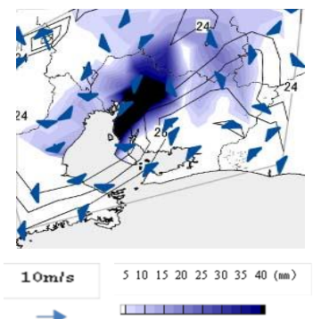
図 - 2 a) - ①に該当する典型事例 (等値線と矢印はそれぞれ海面気温と風向・風速を表す)
