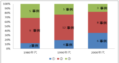
図 - 6 気圧配置による分類の年代別の傾向
