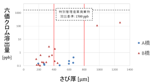
図3 六価クロム溶出量とさび厚の関係
