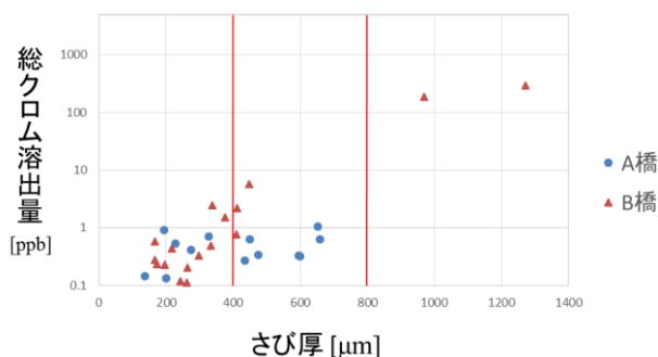
図2 総クロム溶出量とさび厚の関係
