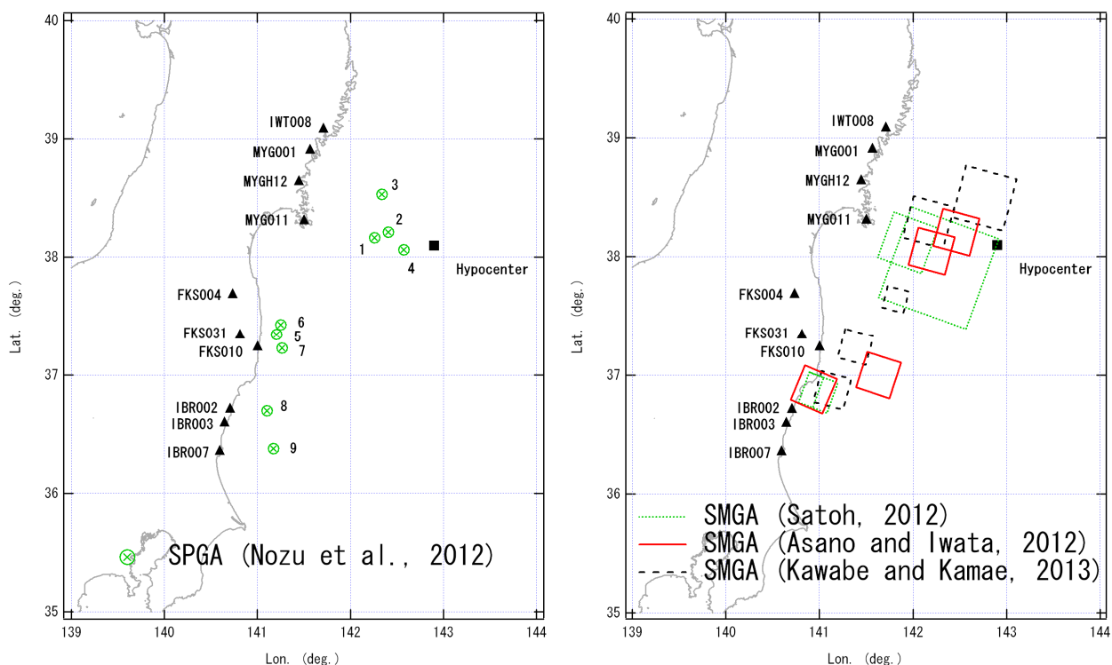
図-1 検討の対象とした震源モデル. (左) SPGA モデル, (右) SMGA モデル.
