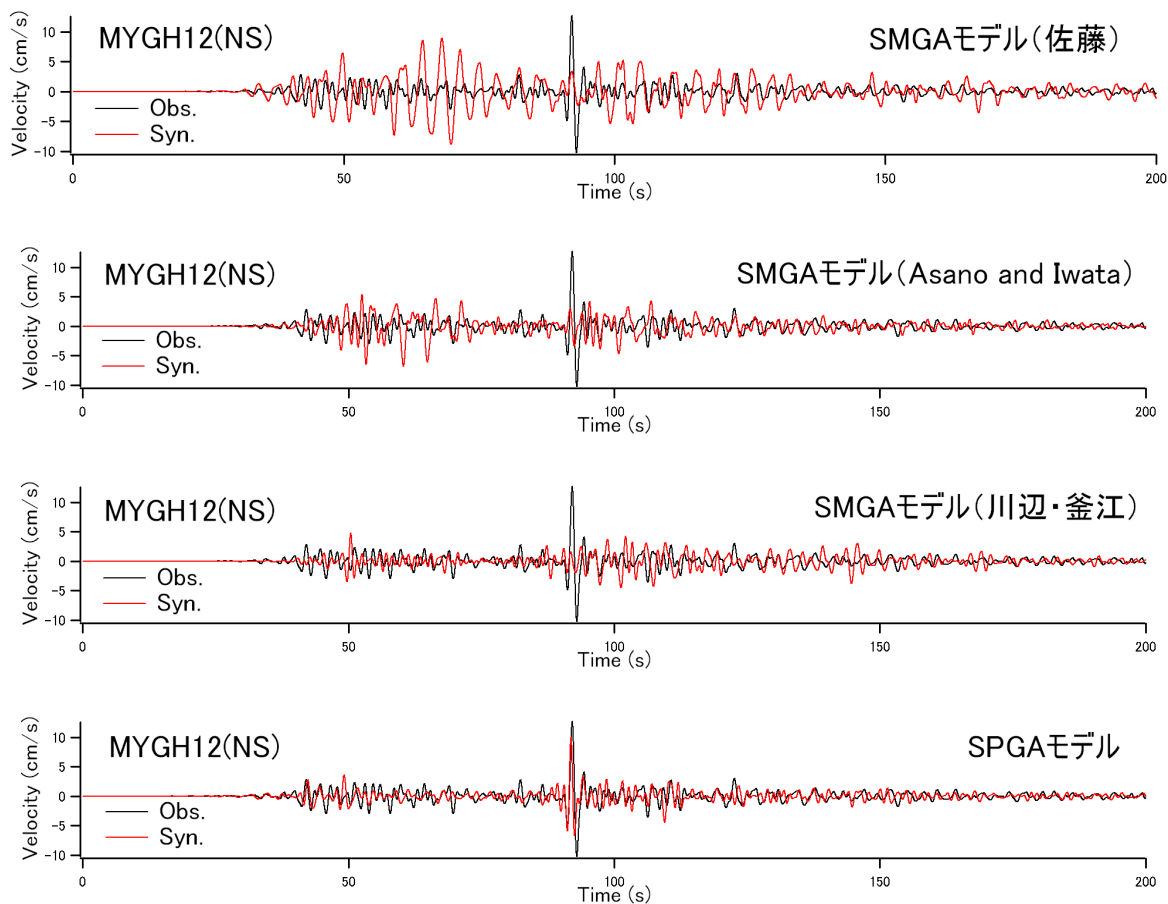
図-2 MYGH12 における速度波形 (0.2-1Hz) の観測結果 (黒) と計算結果 (赤)
