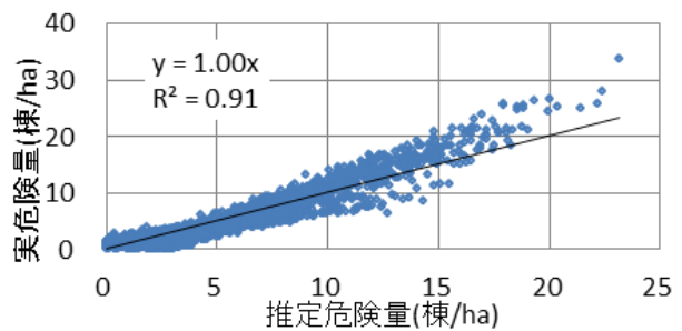
図1 東京都の危険量と推定危険量の関係
