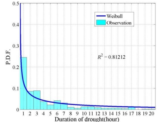
図4 連続無降雨時間の確率密度関数
