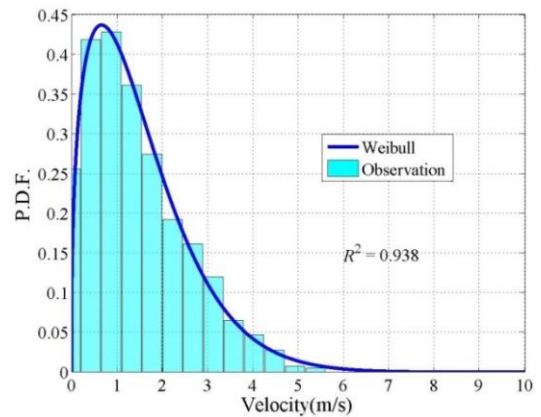
図3 風速の確率密度関数 (WSW)
