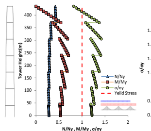
図 11 終局時の側塔 2 塔頂部応力分布
