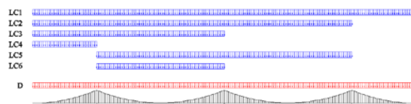
図 7 活荷重载荷条件
