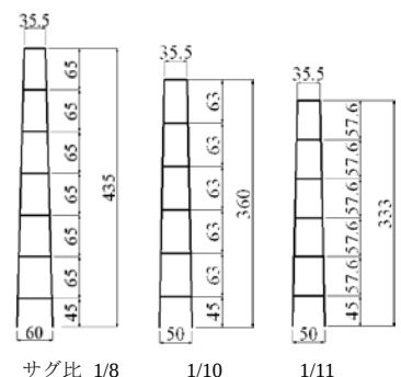
图 2 主塔形状(m)
