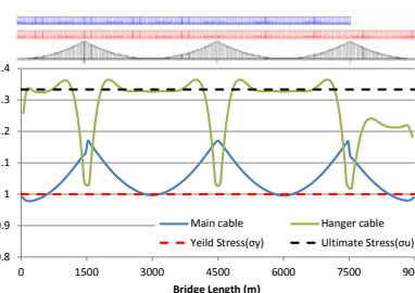
図 12 終局時のケーブル応力分布
