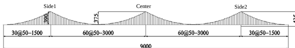
図1 全体形状(サグ比 1/10, (m))
