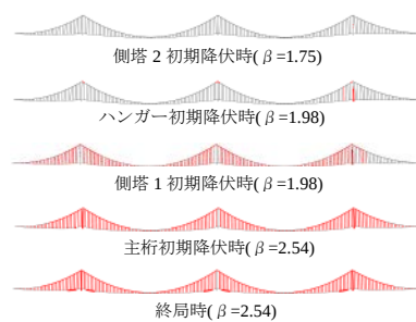
図 10 LC2 における崩壊形状モード
