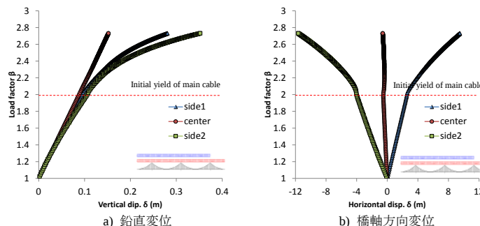
図 13 主塔塔頂部荷重変位曲線 (サグ比 1/8 モデル)
