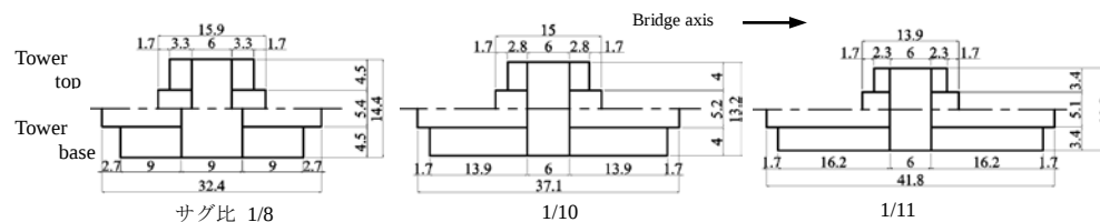
图3 主塔断面 (m)
