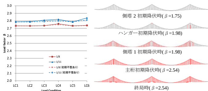
図 9 各モデルの終局時荷重倍率
