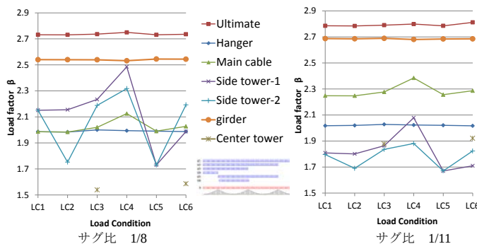
図 8 初期降伏時および終局時の荷重倍率
