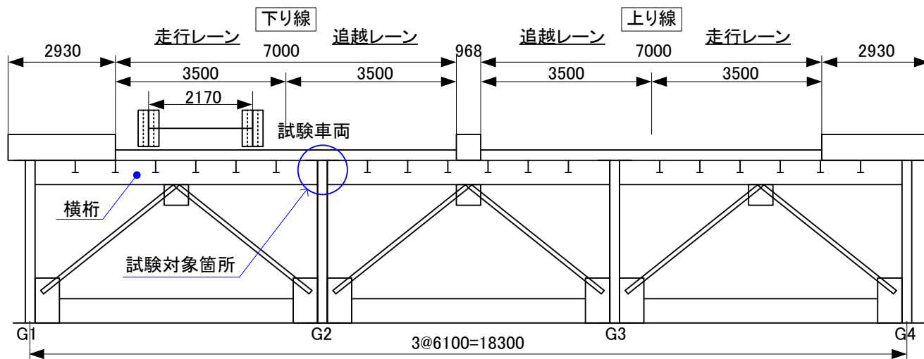
図 3. 実橋の载荷状況
