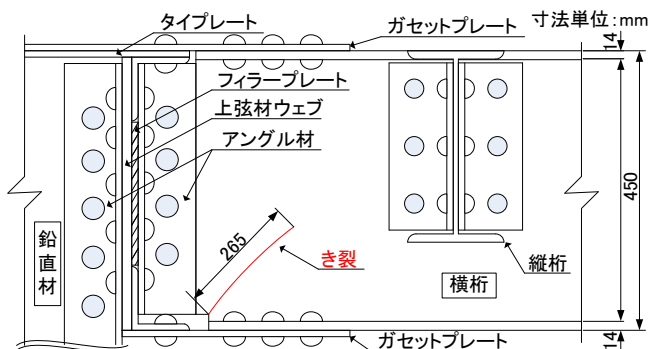
図1. 上弦材と横桁取合い部構造詳細
