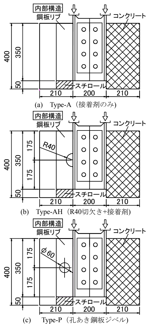
図-1 供試体構造図
