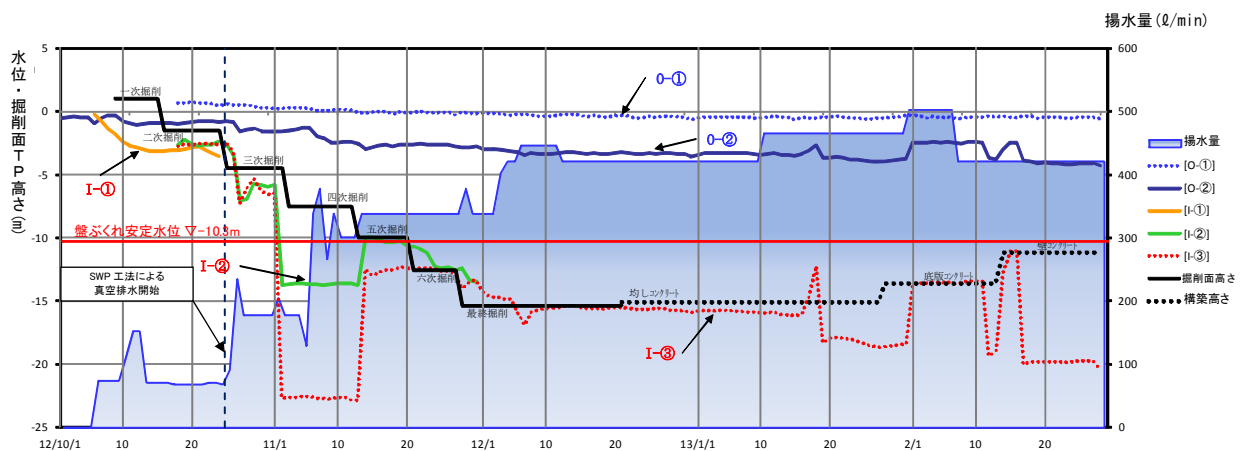
図3 地下水位および揚水量の推移
