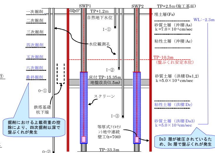
図2 土留め・SWP および掘削断面模式図
