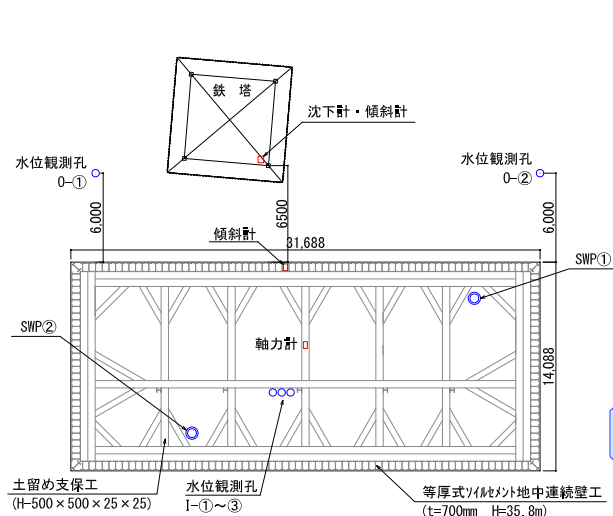
図1 掘削・土留め工平面図
