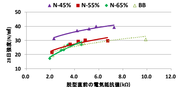
図-7 脱型直前の電気抵抗値と28日強度の関係
