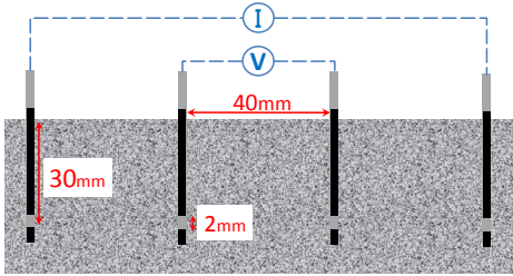
図-2 四電極法概要図
