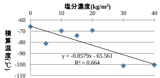
図-3 パッシブ法での積算温度と濃度の関係
