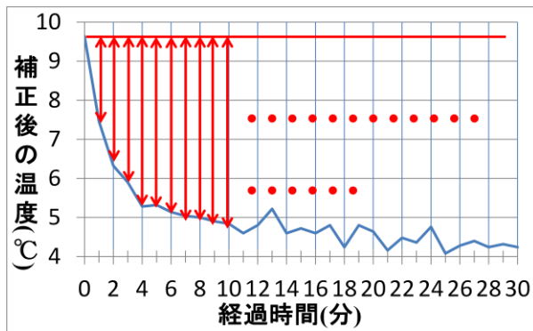
図-1 積算温度の求め方
