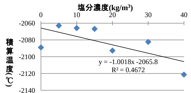
図-4 積算温度と濃度の関係(乾燥炉)
