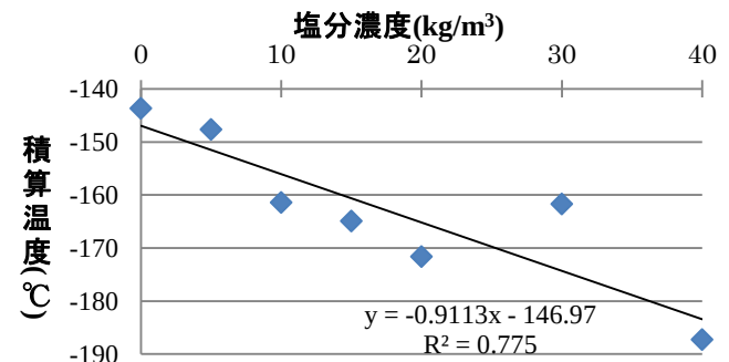
図-2 積算温度と塩分濃度の関係(投光器使用)
