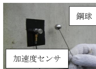
写真-2 インパクトエコー法による計測状況
