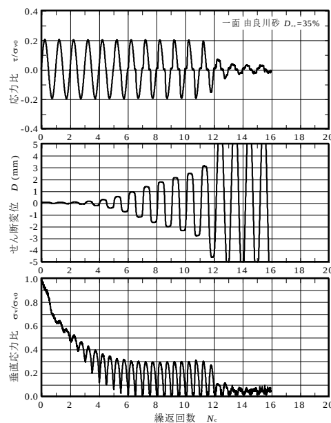
図1 繰返し一面せん断試験結果
