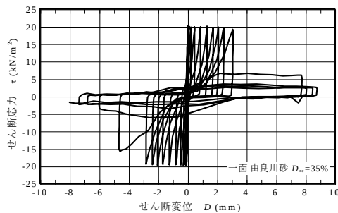
図2 せん断応力-せん断変位関係
