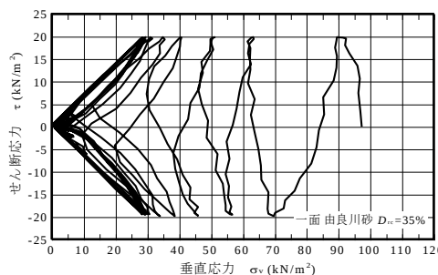
図3 応力経路図
