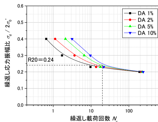
図-4 液状化強度曲線
