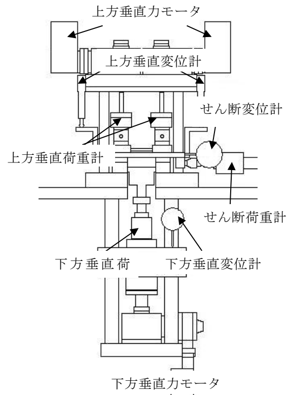
図1 高知高専型一面せん断試験機の概略
