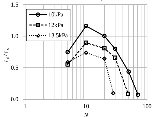
図4 残存強度比( e_0=0.85 )
