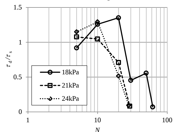
図5 残存強度比( e_0=0.75 )
