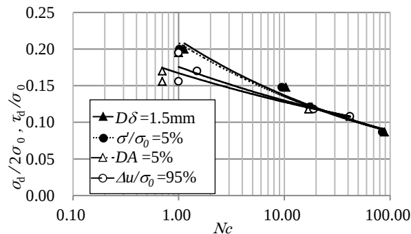
図2 液状化曲線( e_0=0.85 )
