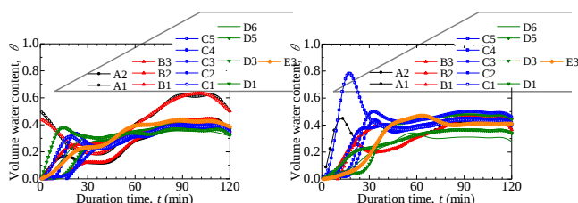
図-4 降雨強度 80mm/hr 時(猛烈な雨)水分量比較, 左: 雨滴小, 右: 雨滴大
