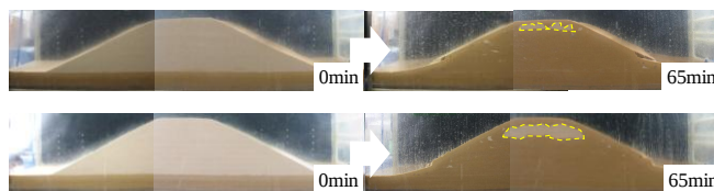
図-1 降雨強度 80mm/hr 時(猛烈な雨)における堤体断面の比較, 上: 雨滴小, 下: 雨滴大
