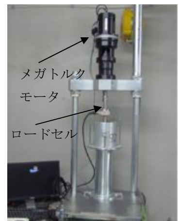
写真1. 試験装置
