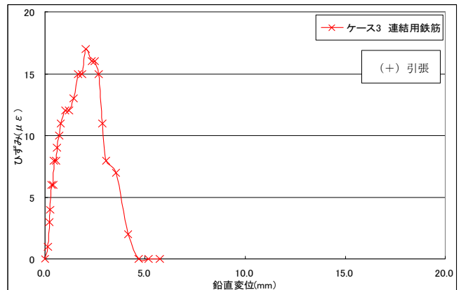
図 - 4 連結用鉄筋のひずみ
