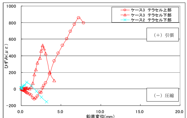
図 - 5 ジオセルのひずみ
