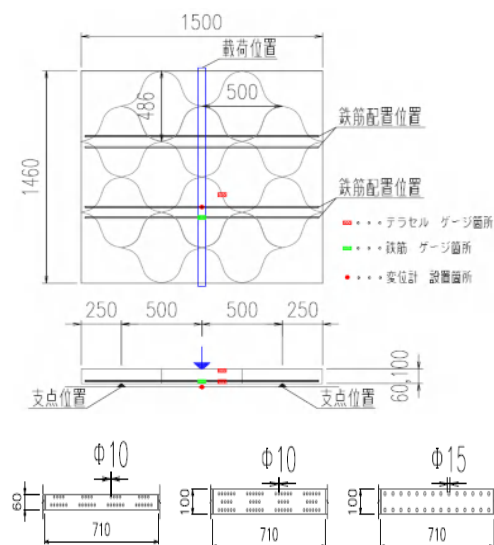
図-1 曲げ試験供試体
