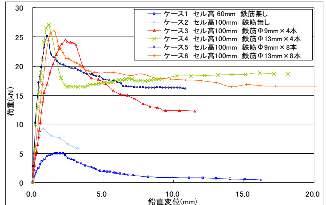
図 - 3 曲げ荷重と鉛直変位の関係
