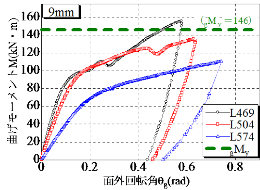
図-2 M - \theta_g 関係
