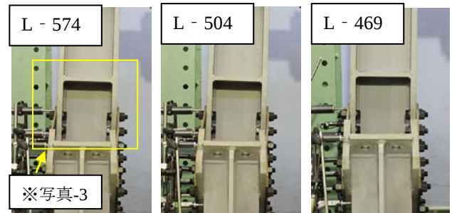
写真-2 ガセットの面外変形状況 (最大荷重作用時)
