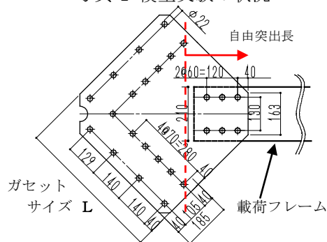
図-1 ガセットの詳細
