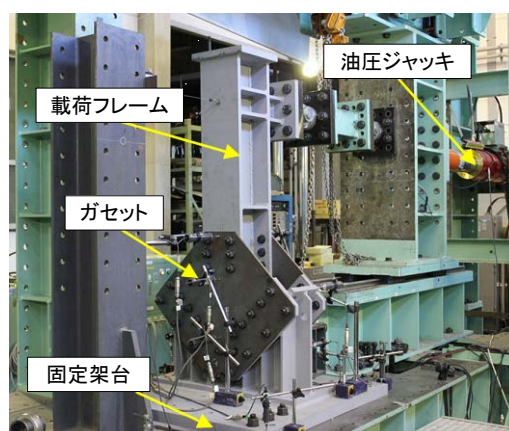
写真-1 模型実験の状況
