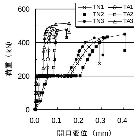
圖-2 荷重-變位曲線
