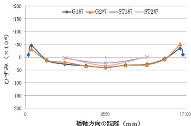
図-3 橋面中央 1 台載荷時の静ひずみ分布
