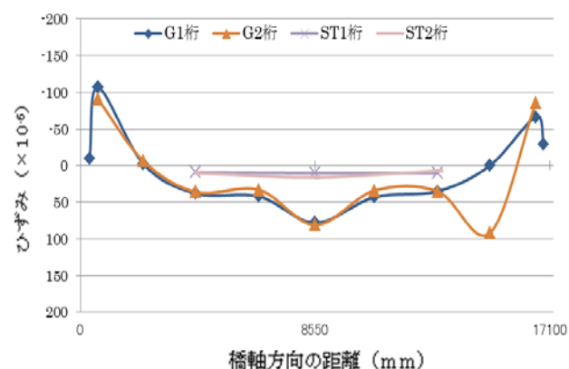
図-4 橋面中央に縦列 2 台載荷時の静ひずみ分布
