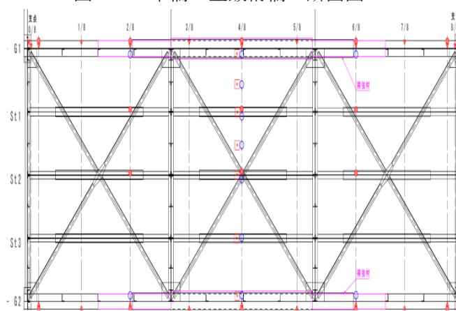
図-2 計測径間のゲージ貼付位置図
