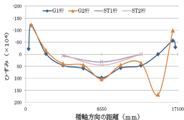
図-5 橋面中央に並列 2 台載荷時の静ひずみ分布
