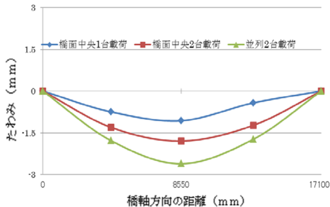
図-7 各載荷パターン時の G_2 桁のたわみ分布
