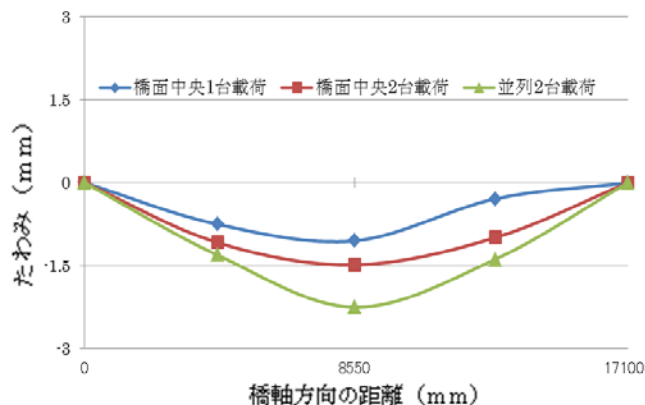
図-6 各載荷パターン時の G_1 桁のたわみ分布
