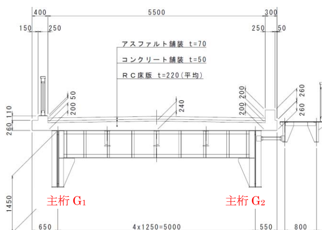
図-1 九年橋 2 主桁桁橋の断面図
