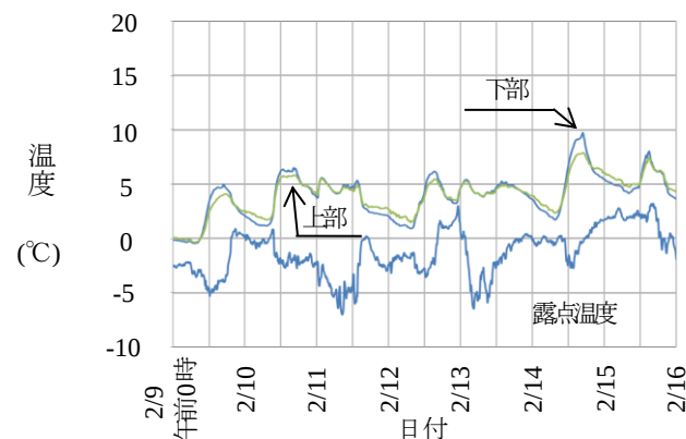
図4 鋼板面温度と露点温度の比較(中央桁)
