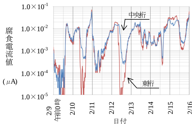
図5 腐食電流値の比較
