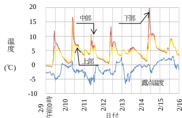
図3 鋼板面温度と露点温度の比較(東桁)
