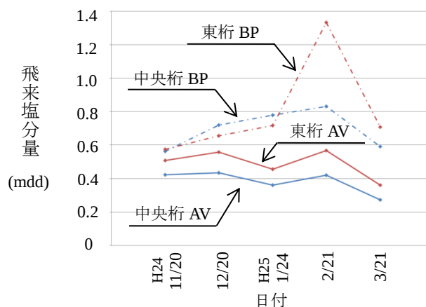
図2 飛来塩分量(曝露期間毎)
