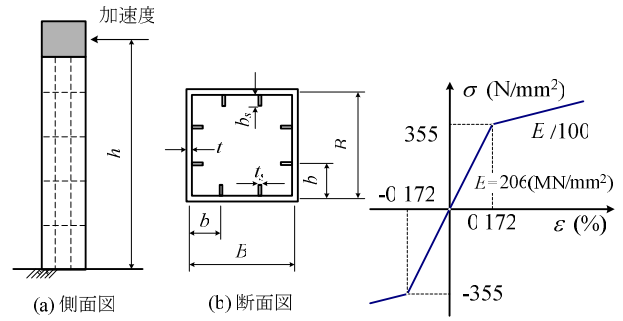
図 1 解析対象モデル 図 2 鋼板の \sigma - \epsilon 曲線
