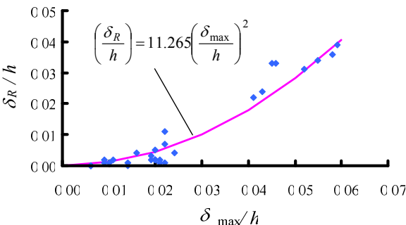
図4 最大応答変位と残留変位の関係
