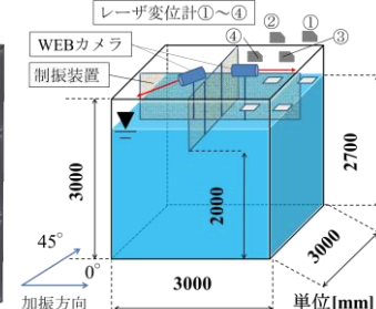
図-2 機器設置図
