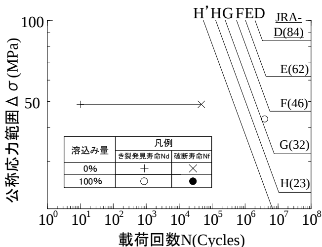
図 5. 溶込み量 0%および 100%試験体の S-N 線図
