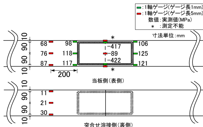
図 3. 溶込み 0%試験体の応力分布
