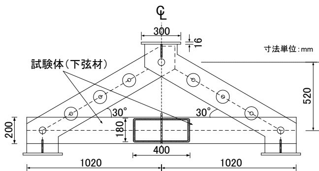
図 2. 載荷冶具の形状と寸法
