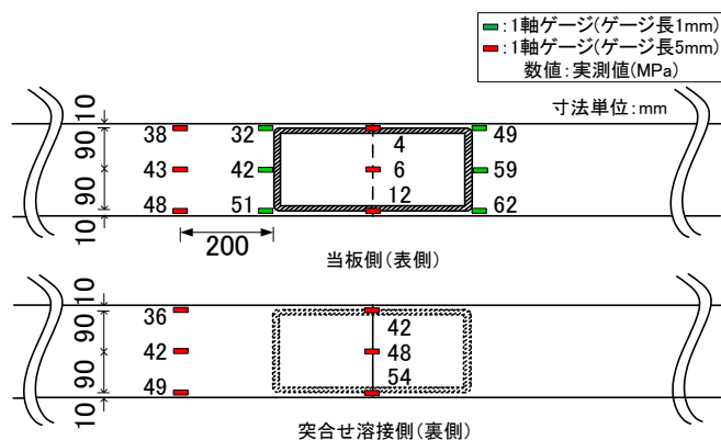
図 4. 溶込み 100%試験体の応力分布
