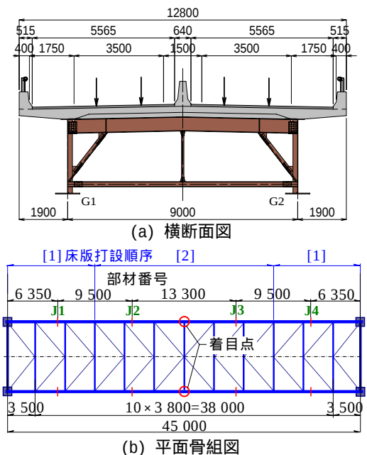
図-1 計算対象の単純合成桁モデル
