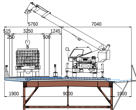
(b) 床版鋼材パネルの敷設
