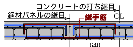
図-3 床版の継目位置
