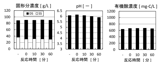
図-2 水熱処理条件の検討の実験結果（実験 II）
