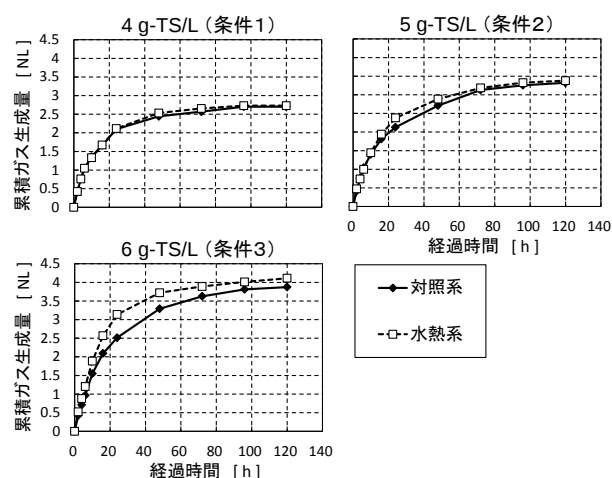
図-4 累積ガス生成量の経時変化
