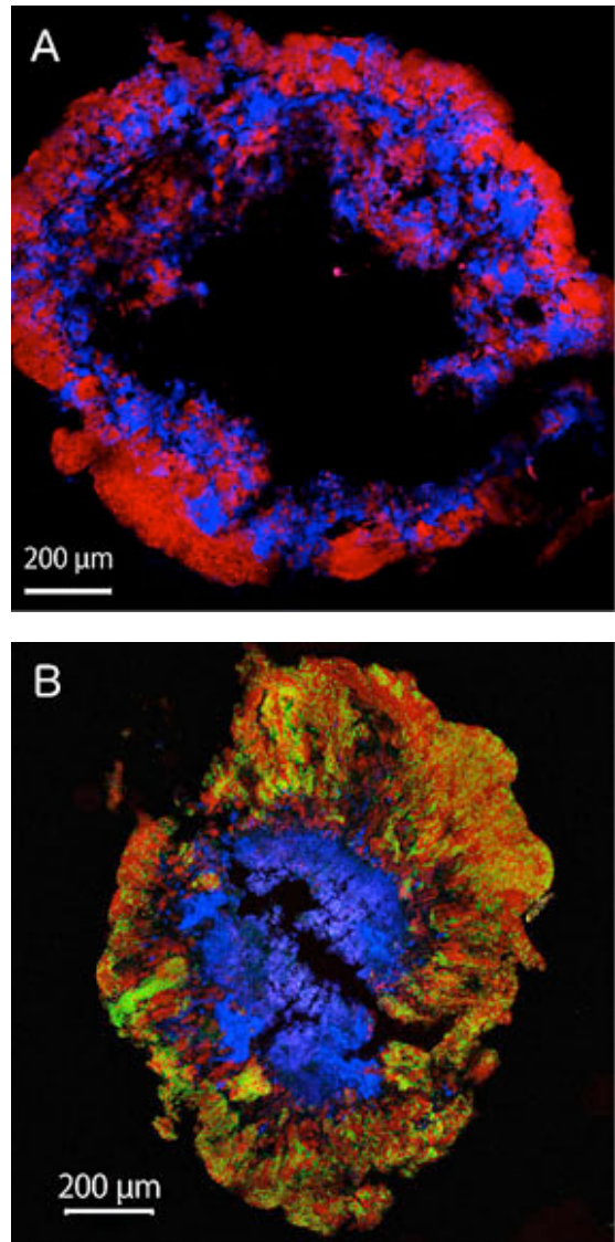
図2. 多重染色FISH法によるグラニユール汚泥微生物群集の空間構造. A: EUB338 (赤) と ARC915 (青), B: Syntrophorhabdaceae 科 (青), Cryptanaerobacter 属 (緑), Syntrophus 属 (赤).
