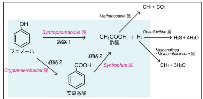
図1. 16S rRNA 遺伝子に基づくクローン解析結果から想定される UASB グラニュール汚泥内でのフェノール分解経路
