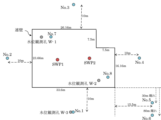
図 1 平面図
