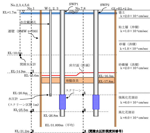
図 2 断面模式図
