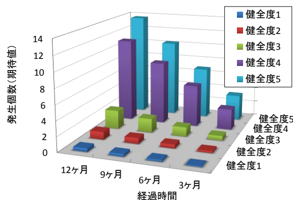
図-3 ポットホール発生個数の期待値
