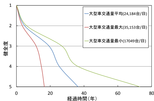
図-1 ひび割れの期待劣化曲線
