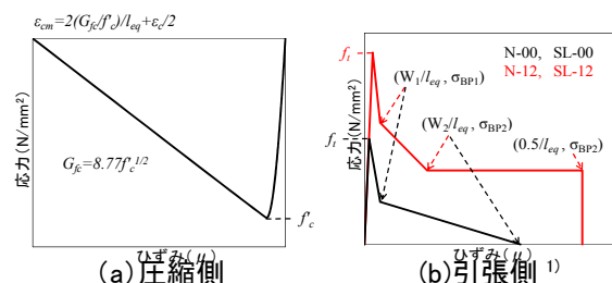
図-2 使用したコンクリートの材料構成則
