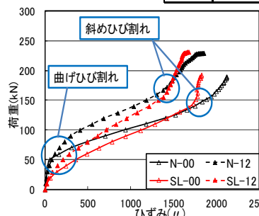
図-5 荷重-鉄筋ひずみ関係
