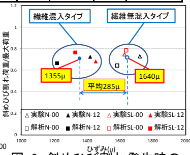
図-6 斜めひび割れ発生時の鉄筋ひずみ差
