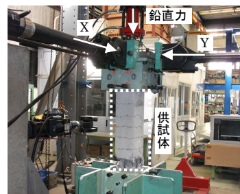
写真-1 二軸載荷装置
