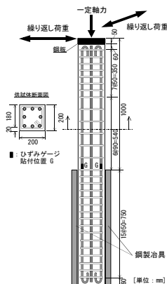
図-1 供試体配筋図
