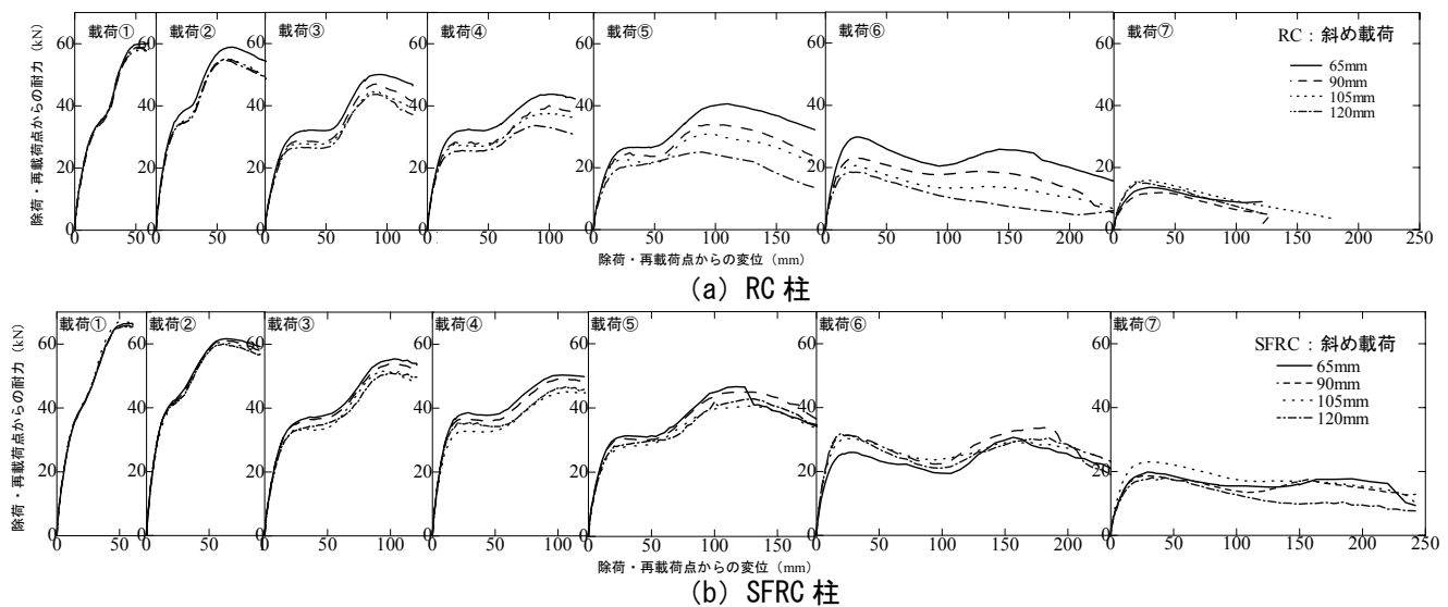
図-5 耐力-変位関係 ( f'_{ck} = 60 \text{ MPa} の場合)
