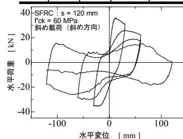
(b) SFRC 柱
