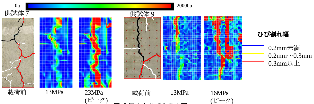
図-5 最小主ひずみ分布図
