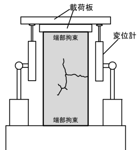
図-1 載荷試験の状況
