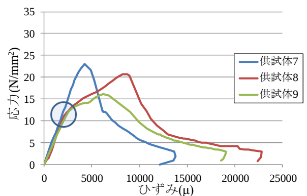
図-4 応力-ひずみ関係（端部拘束無）
