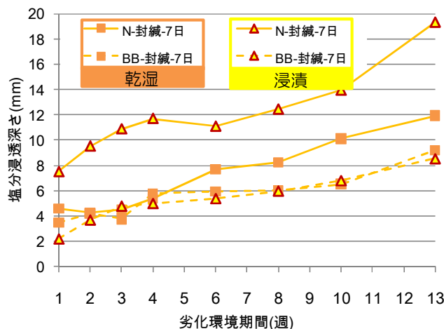
図-2 セメント種類と塩分浸透深さの関係
