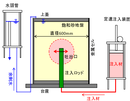
図-1 注入装置の模式図
