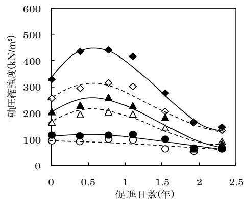
◆: 水ガラス濃度 25%, ▲: 水ガラス濃度 19%, ●: 水ガラス濃度 12.5% 相対密度 80% 相対密度 80% 相対密度 80% ◇: 水ガラス濃度 25%, △: 水ガラス濃度 19%, ○: 水ガラス濃度 12.5% 相対密度 60% 相対密度 60% 相対密度 60%
