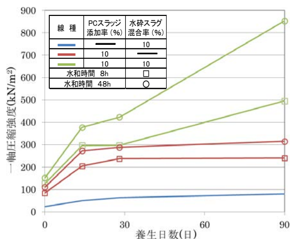
図－3 養生日数と一軸圧縮強度
