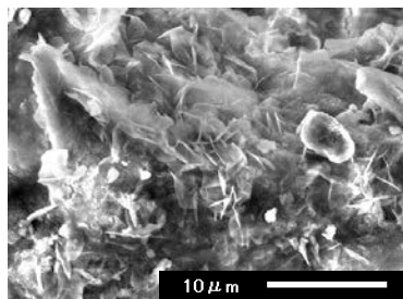
(b) 改良土中の水砕スラグ (養生 1 日)
