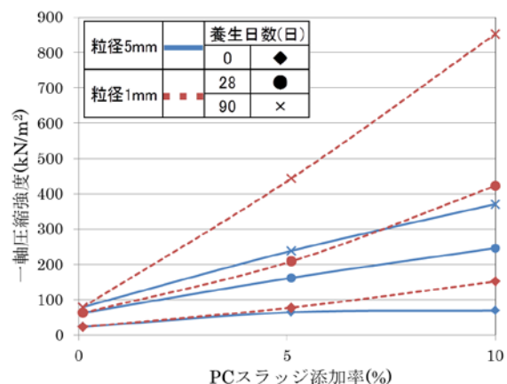
図－2 PC スラッジ添加率と一軸圧縮強度 (最大粒径 1mm、水和時間 8h、水砕スラグ 10%)
