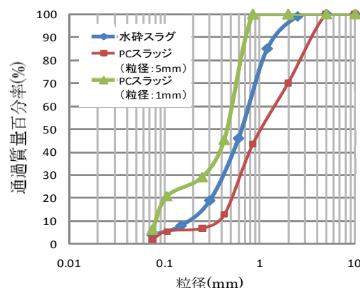
図-1 PC スラッジ、スラグの粒度分布
