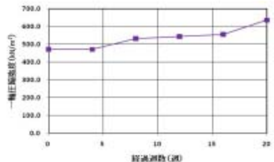
図4.一軸圧縮強度と経過週数の関係
