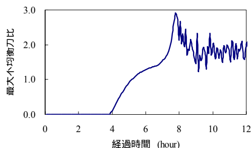
図-3 最大不均衡力比の経時変化
