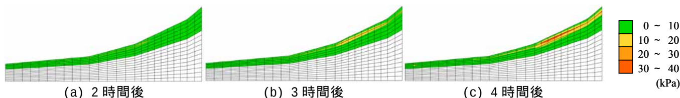
図-8 間隙空気圧分布の経時変化
