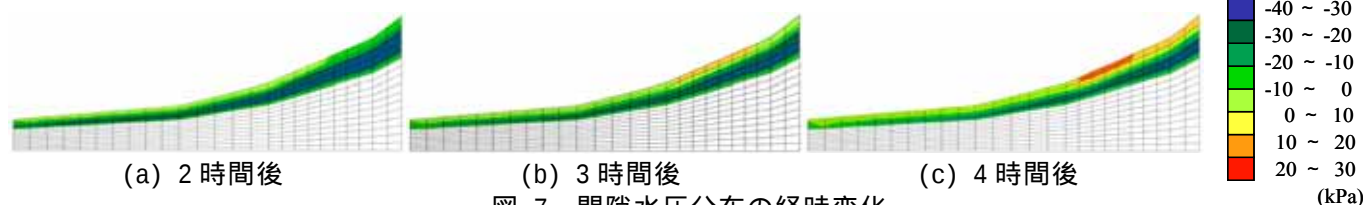
図-7 間隙水圧分布の経時変化
