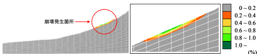
(a) 全体図 (b) 崩壊部周辺 図-6 せん断ひずみ増分分布図(4 時間後)
