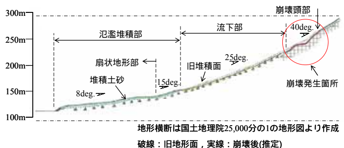
図-1 福智町斜面崩壊の縦断図(推定) 1)
