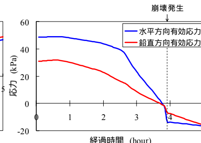
図-5 有効応力の変化
