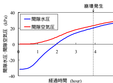
図-4 間隙圧の変化
