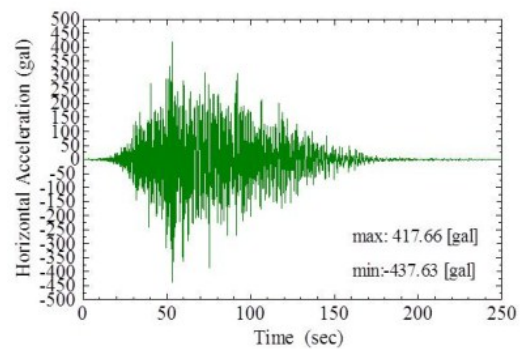
図2 入力地震動
