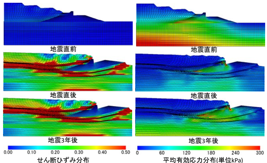
図3 せん断ひずみ分布と平均有効応力分布
