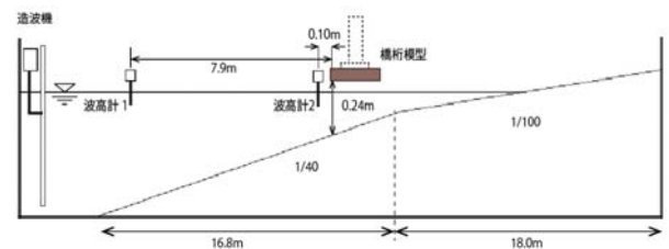
図1 実験装置の概要(長方形断面)
