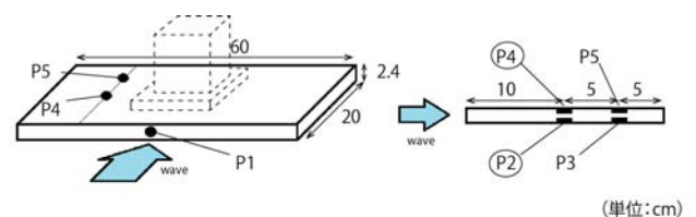
図2 橋桁模型と波圧測定点 (単位:cm)
