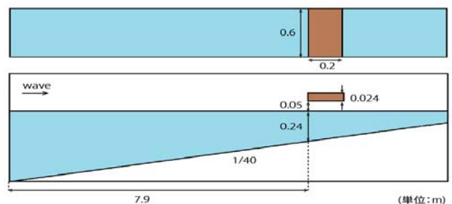
図3 解析領域の概要(長方形断面) (単位:m)
