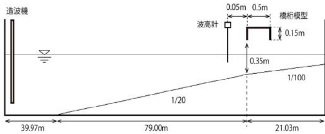
図6 実験装置の概要(溝形断面)
