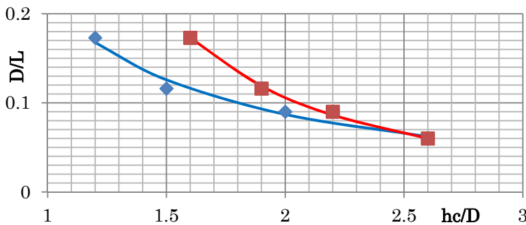
図2 V_d/V_0=1.2 となるための D/L と hc/D との関係 ■ : Case A ◆ : Case B
