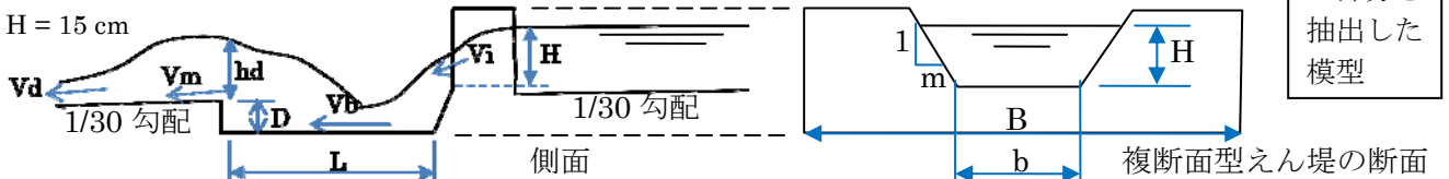
図1 掘り込み型減勢工の定義図
