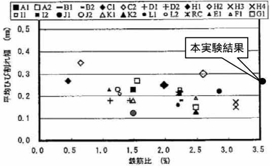
図 - 4 ひび割れ幅の比較 ( \sigma_s=140\text{N/mm}^2 )
