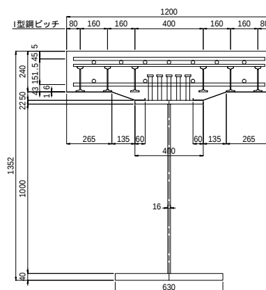
図 - 1 供試体断面図
