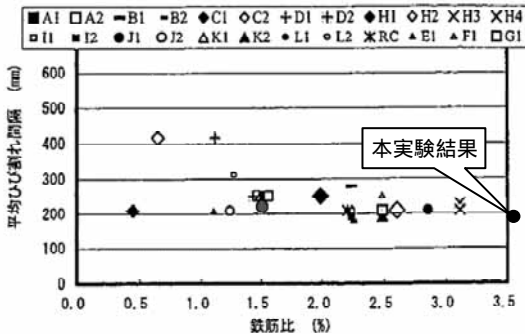
図 - 3 ひび割れ間隔の比較 ( \sigma_s=140\text{N/mm}^2 )
