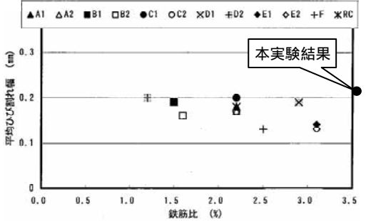
図 - 5 ひび割れ幅の比較 ( \sigma_s=120\text{N/mm}^2 )
