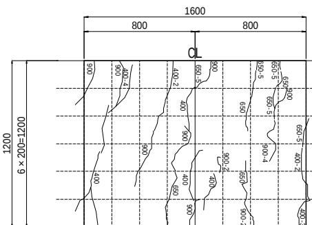
図 - 2 ひび割れ発生状況図
