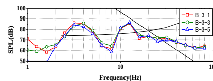
Fig.2.2 低周波音圧レベル(B-3 南行)
