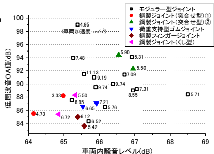
Fig.7 車両内騒音—低周波音 OA 値
