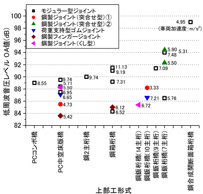
Fig.8 上部工形式—低周波音 OA 値
