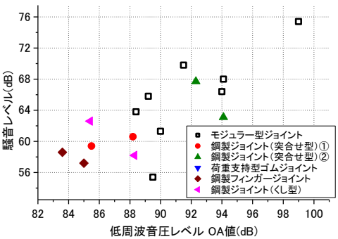
Fig.1 低周波音 OA 値-騒音レベル
