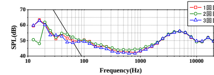
Fig.6.2 通常時車両内騒音
