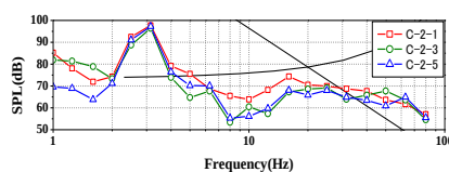
Fig.2.1 低周波音圧レベル(C-2 南行)
