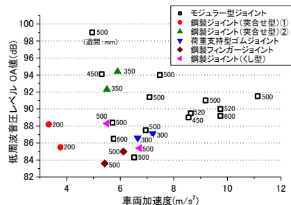
Fig.5 車両加速度—低周波音 OA 値
