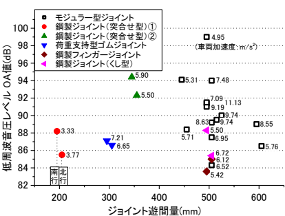
Fig.4 ジョイント遊間量—低周波音 OA 値
