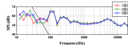
Fig.6.1 B-3 南行通過時車両内騒音
