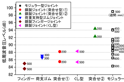
Fig.3 ジョイント形式—低周波音 OA 値
