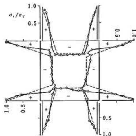
図1 箱形断面部材の一般的な残留応力分布 3)
