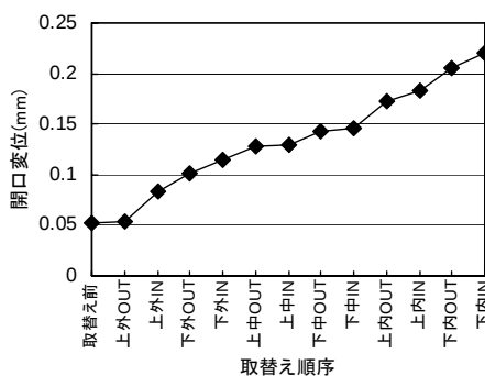
図 3. 開口変位
