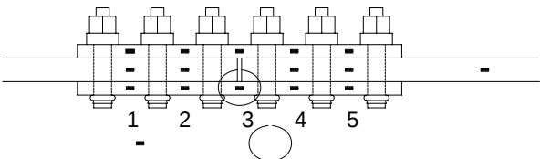
ひずみゲージ クリップゲージ
