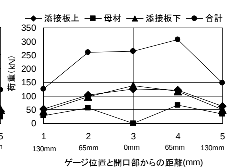
図 5. ボルト取替え後(ケース 5)
