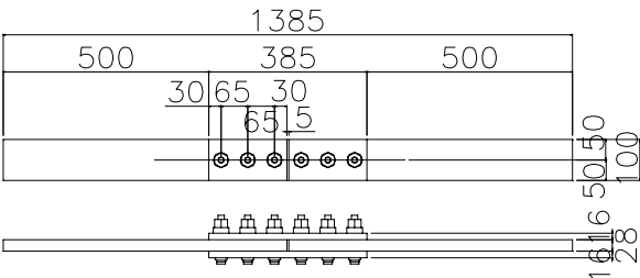
図 1. 試験体形状
