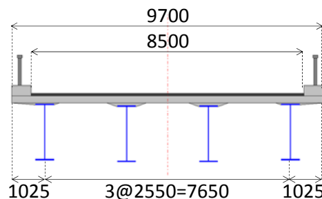
図-3 橋梁の断面(支間長 30m)
