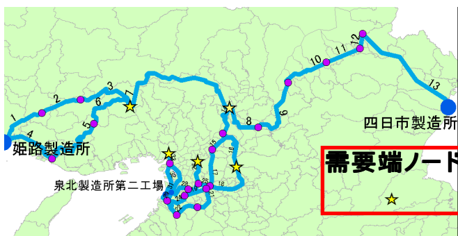
図2 ガス導管システム概略図
