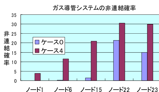
図6 シナリオ地震による非連結確率
