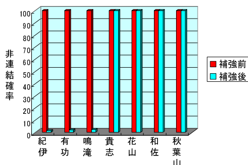
図5 補強前後の非連結確率(津波 5m)
