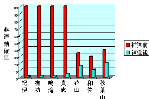
図4 補強前後の非連結確率(津波 3m)
